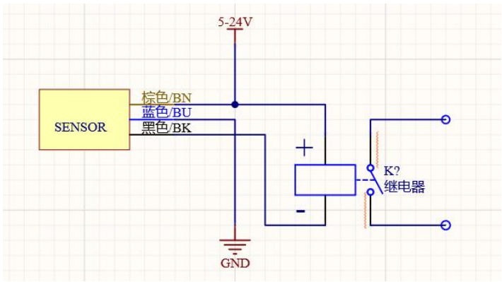
PNP型
